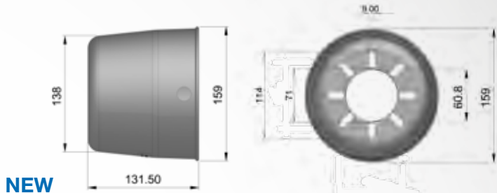
CONTROCUFFIA CILINDRICA CON COLLARE Cylindrical shaft cone with collar
