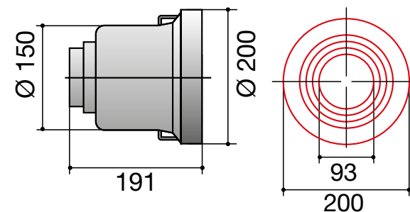
CATENA PER COPERCHI Lid chain
